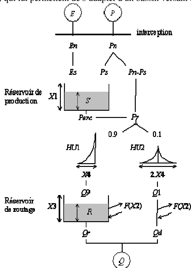
Figure 1 - Schéma du fonctionnement du modèle GR4J
